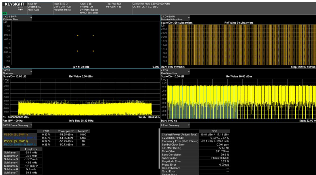
Figure 9. NR V2X demodulation analysis
